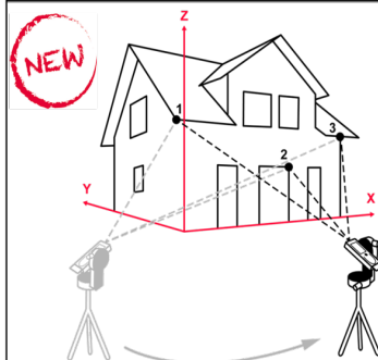
Fonction de relocalisation : déplacement de la station de mesure
