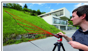
Différence de hauteur
