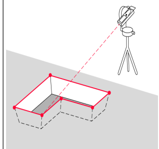
Calcul de volume
