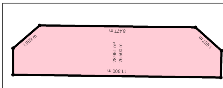
Relevé d'une toiture en 2D
