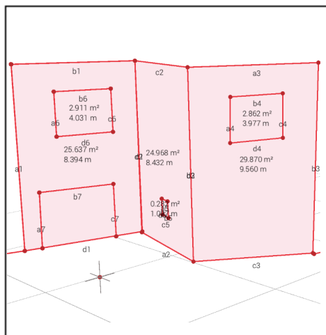
Relevé de façade en 3D
