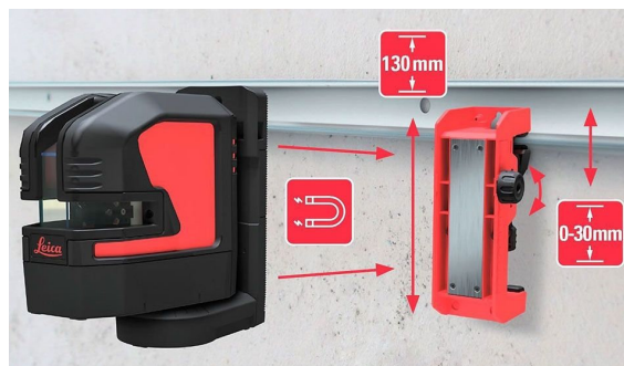
UAL130 wandklem met hoogte instelling tot 130 mm
