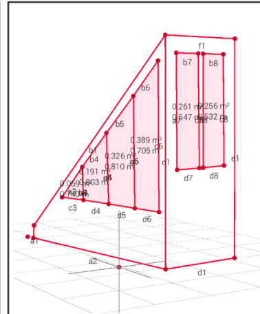
Opmeting ondertrap
