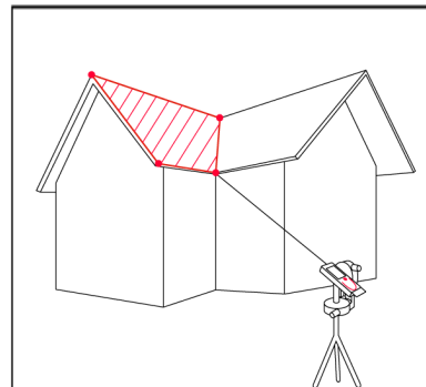
Smart oppervlakte meting van een dak met de Plan App
