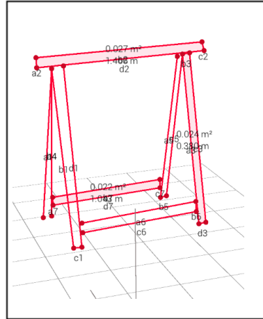
3D meting van een schraag
