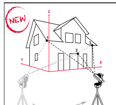
Relocationfunctie: meetstation verplaatsen
