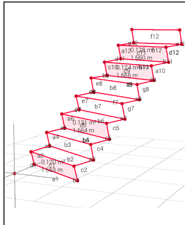
Opmeting trap
