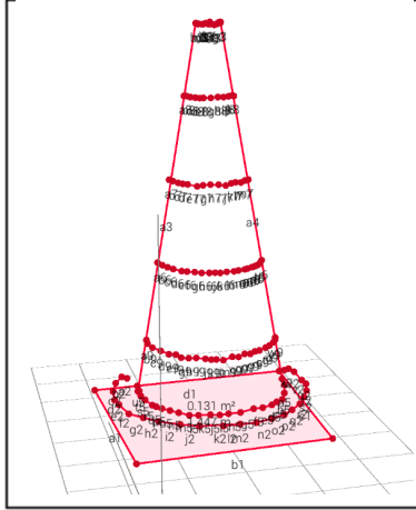
3D meting van een verkeerskegel
