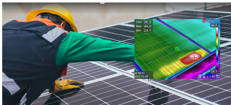
Opsporen defecte cellen van zonnepanelen
