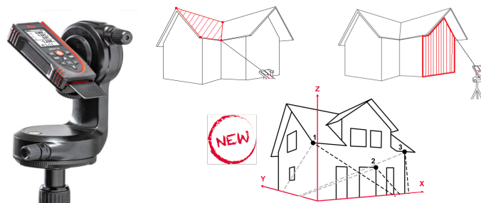
Extensible de manière modulaire avec le kit Disto P2P
