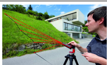
Mesure de différence de hauteur
